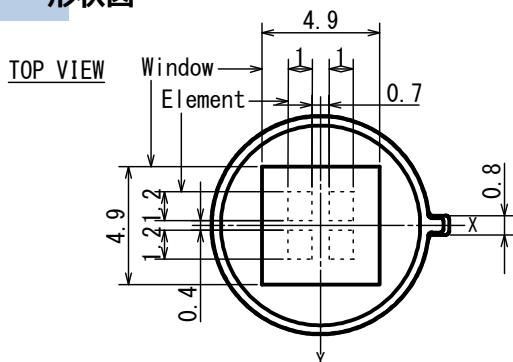
形状図
